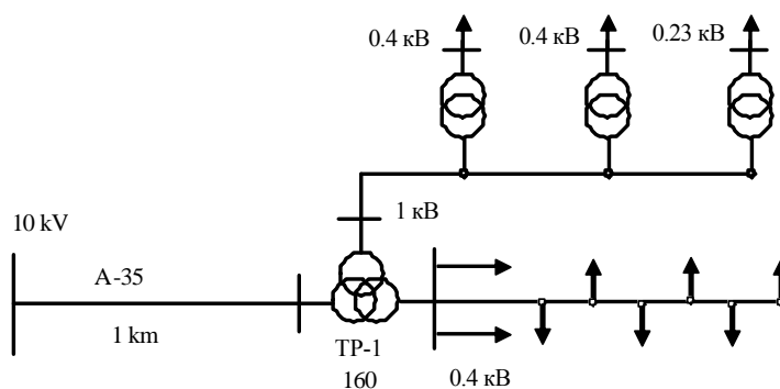
Рис.2. Комбинированные распределительные сети 0.4 кВ с сетью 0.66-1 кВ
