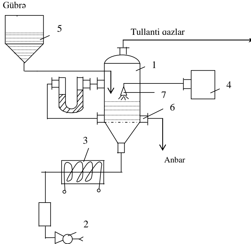
Şəkil 1. Qaynar lay aparatı. 1-qaynar lay aparatı; 2-ventilyator; 3-qızdırıcı; 4-polimer məhlulu üçün tutum; 5-kapsullaşmamış gübrə dənələri üçün tutum; 6-kapsullaşdırılmış dənələrin xaric olması üçün ştuser; 7-çiləyici.
